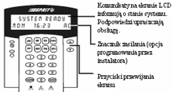
Rys. 1.2. Klawiatura Esprit+ 642 LCD
